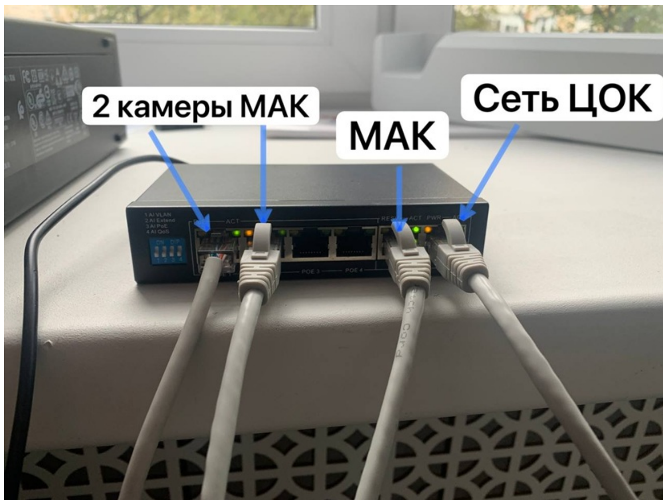
Корректное подключение коммутатора.
